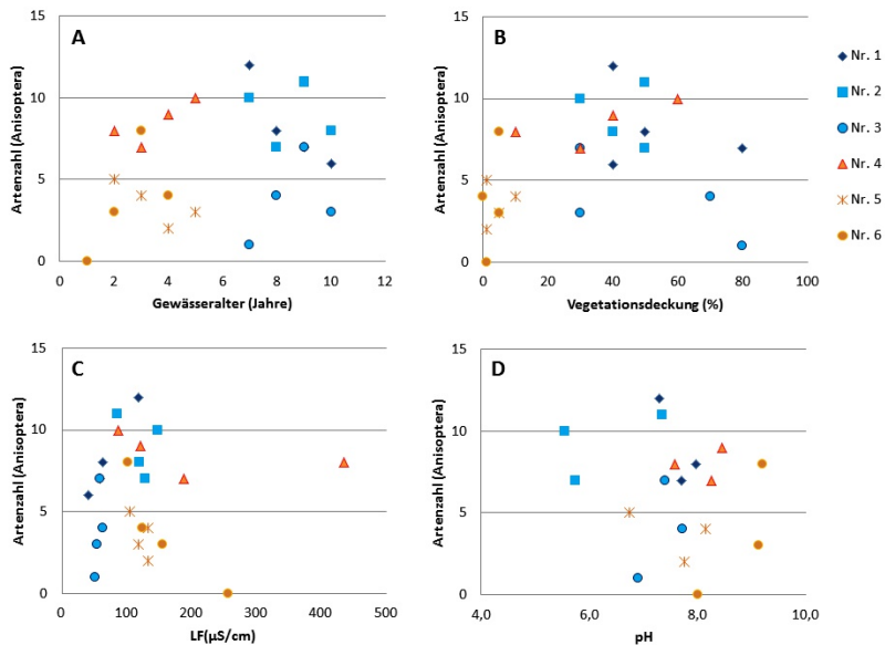
Abb. 5. Zusammenhänge zwischen der Artenzahl der Anisoptera und dem Gewässeralter (A), der Vegetationsdeckung (B), der Leiffähigkeit (C) und den pH-Werten (D).
